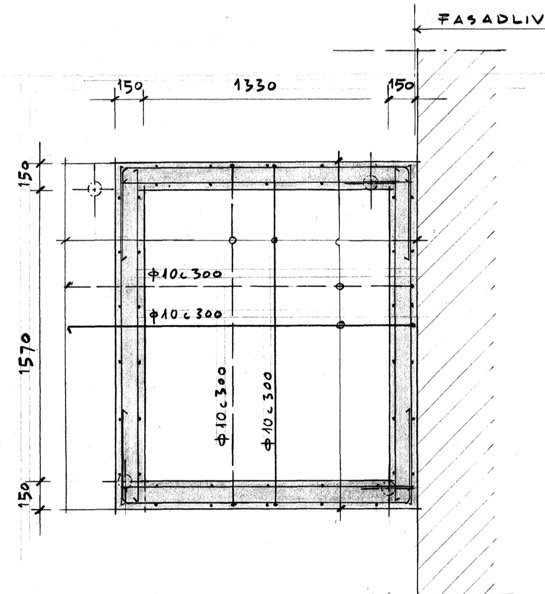
GRUNDPLAN 1:20
