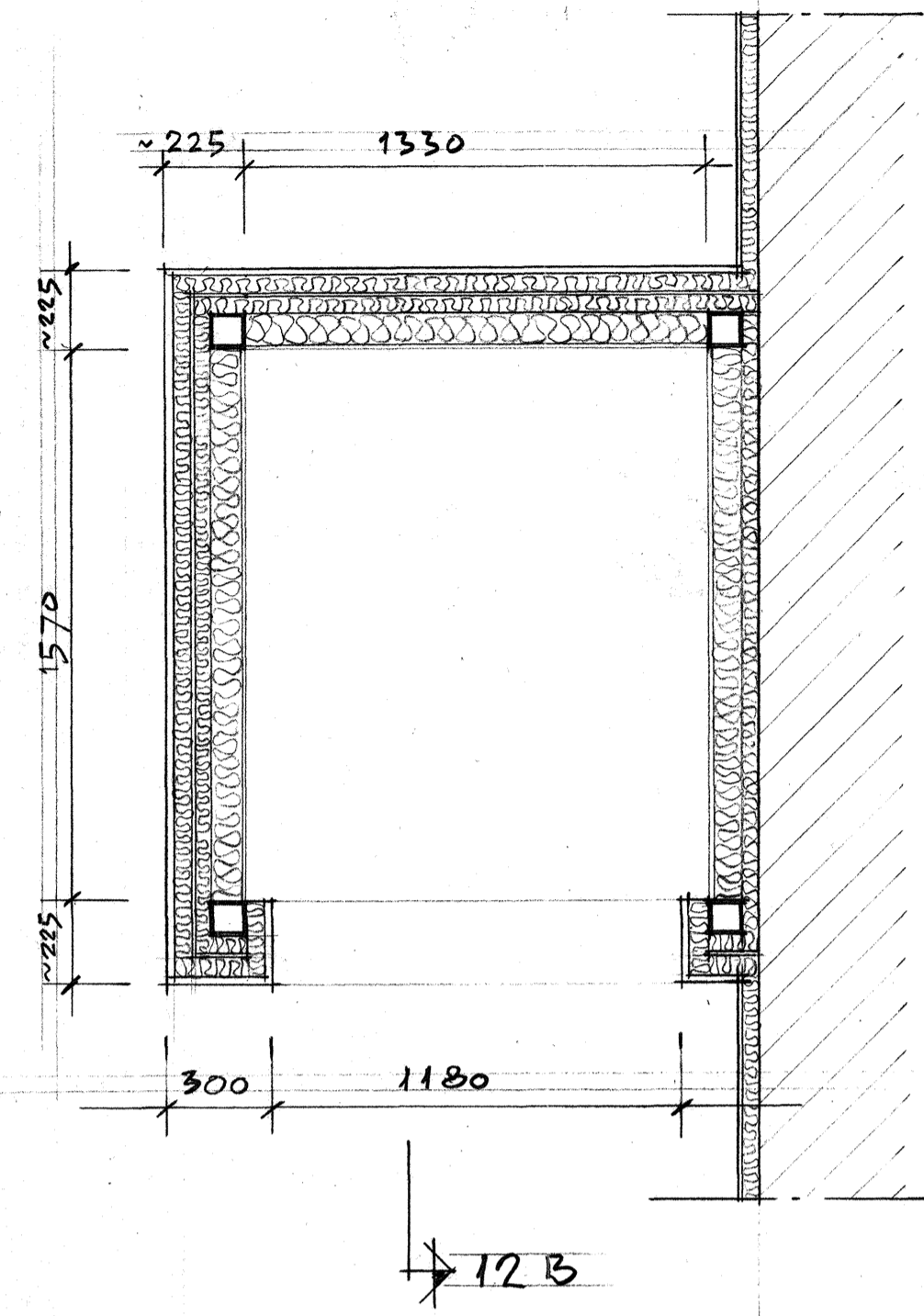
PLANER 1:20
