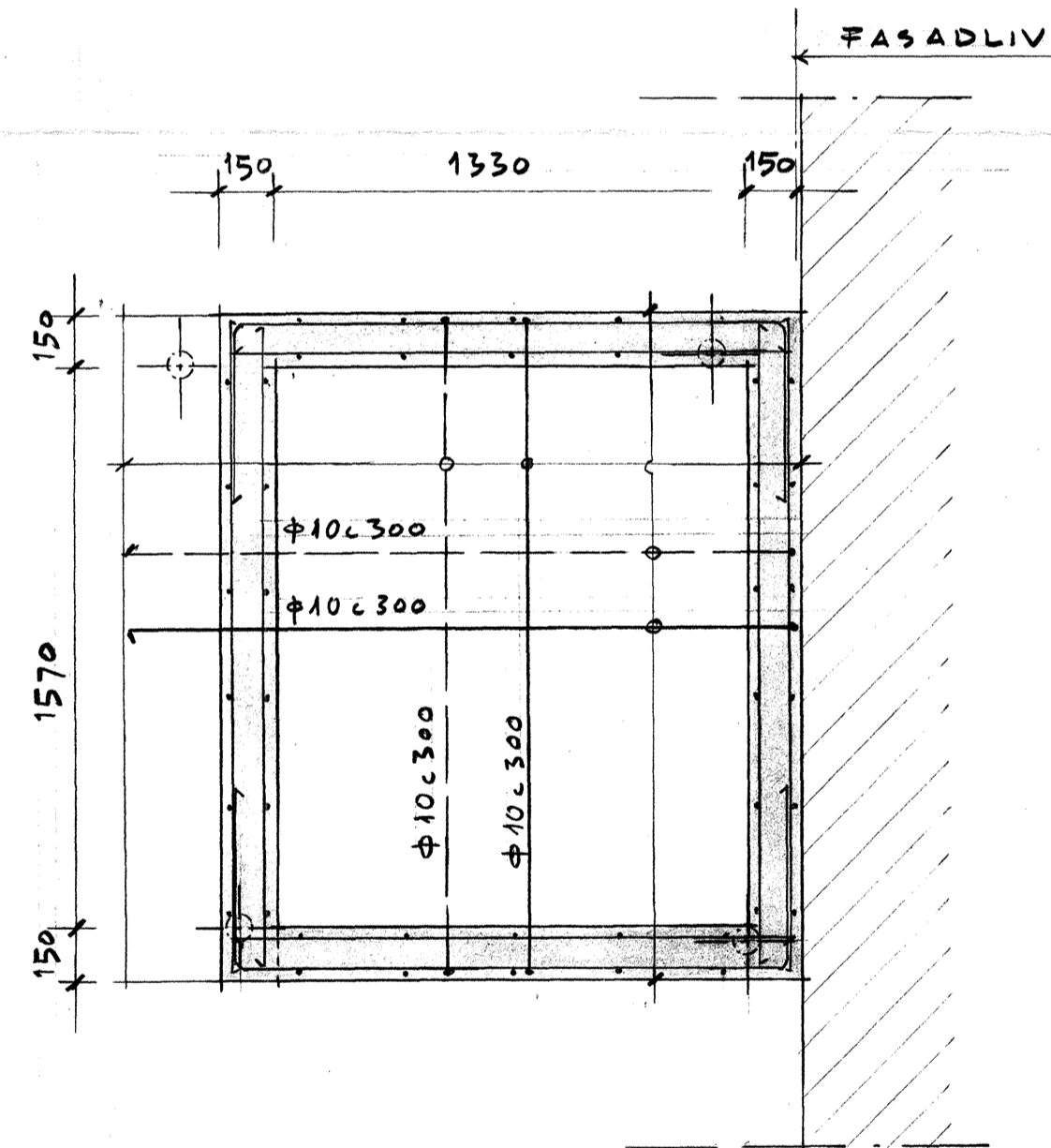
GRUNDFLAN 1:20
