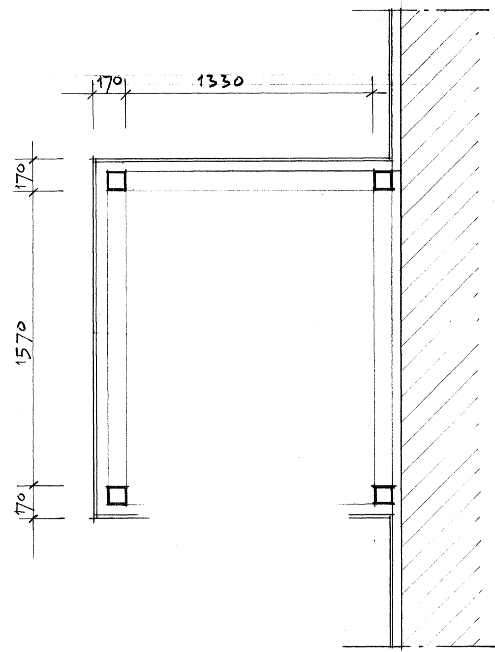
PLANER 1:20
