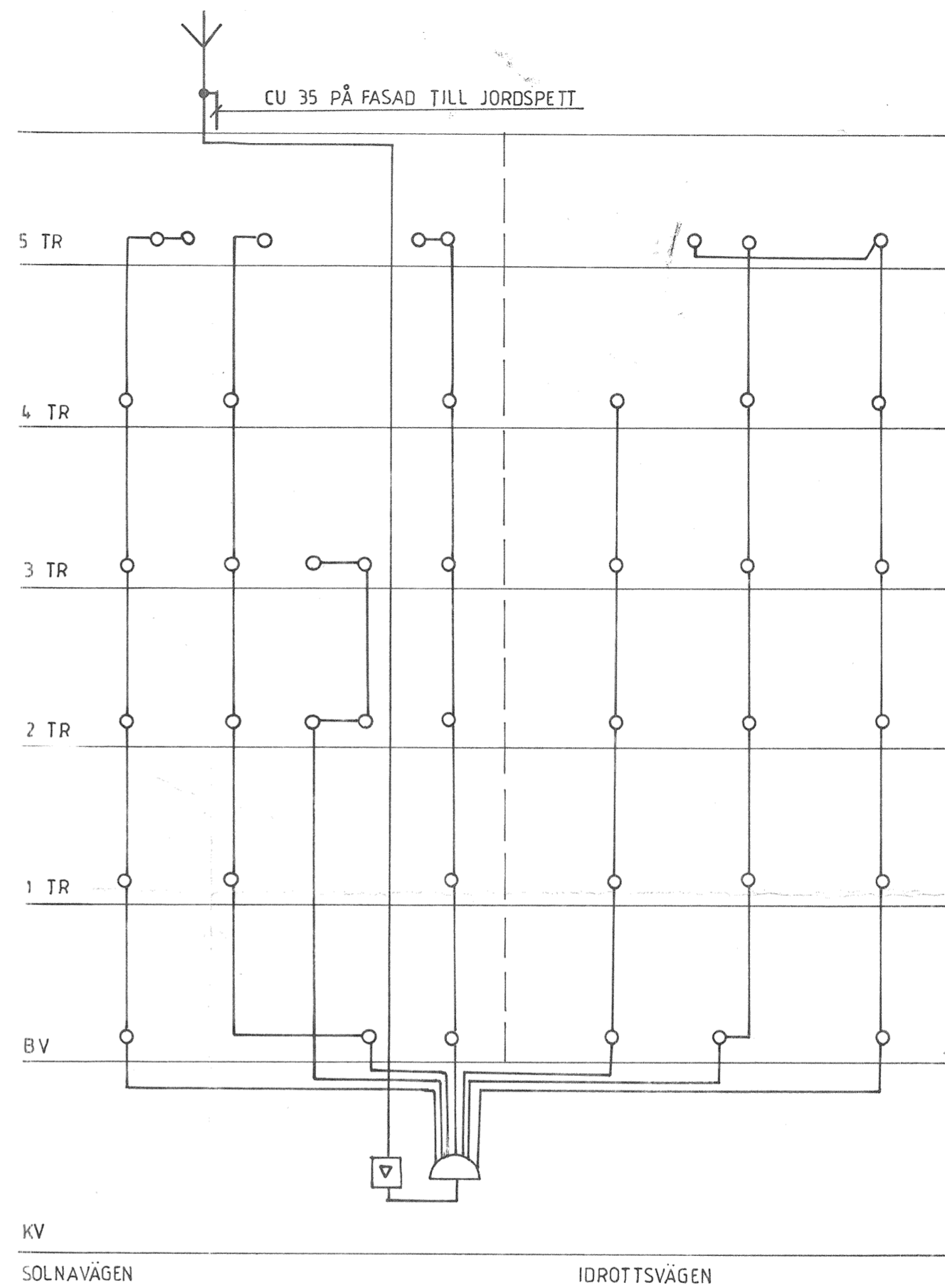
CENTRALANTENNSCHEMA
