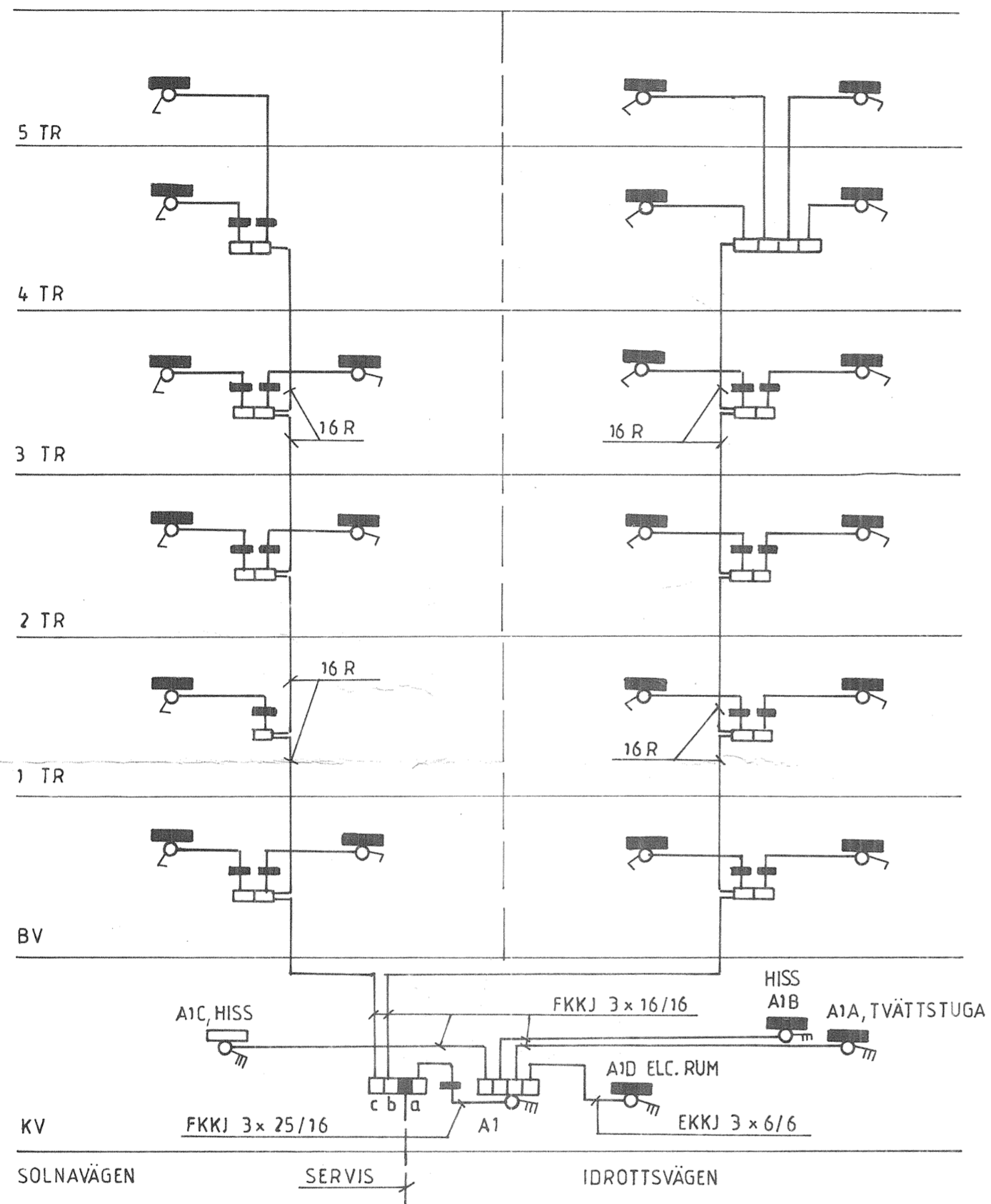
HUVUDLEDNINGSSCHEMA
